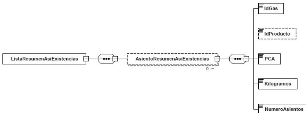
7. irudia. Izakinen laburpen datuak.
