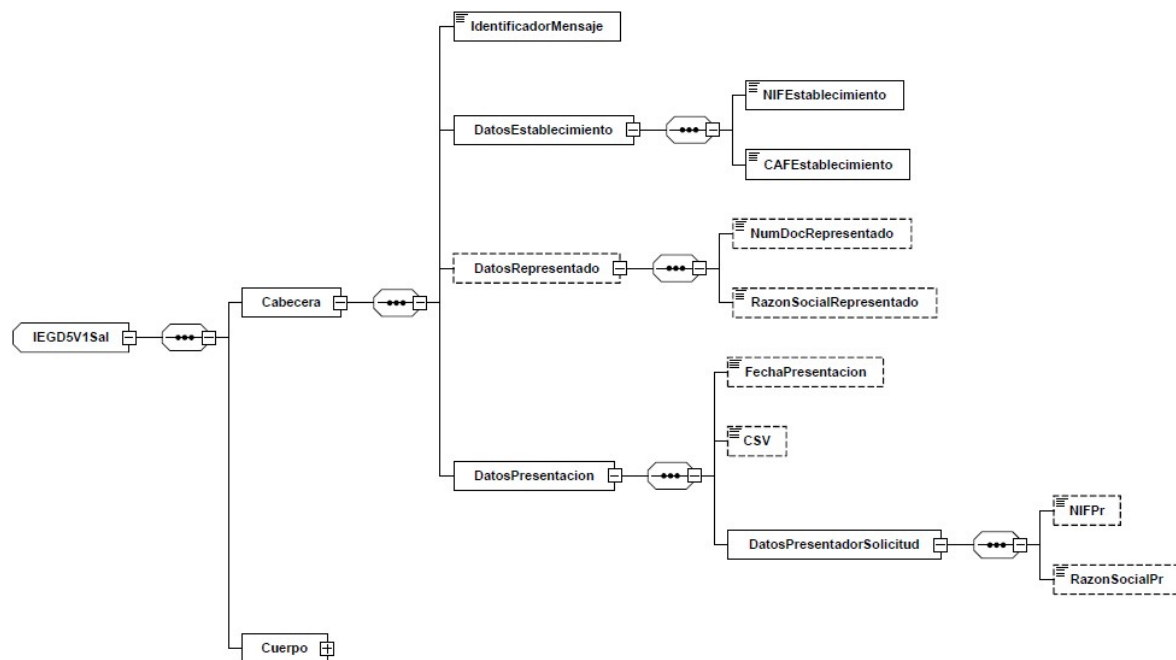
5. irudia. Irteerako mezua.
