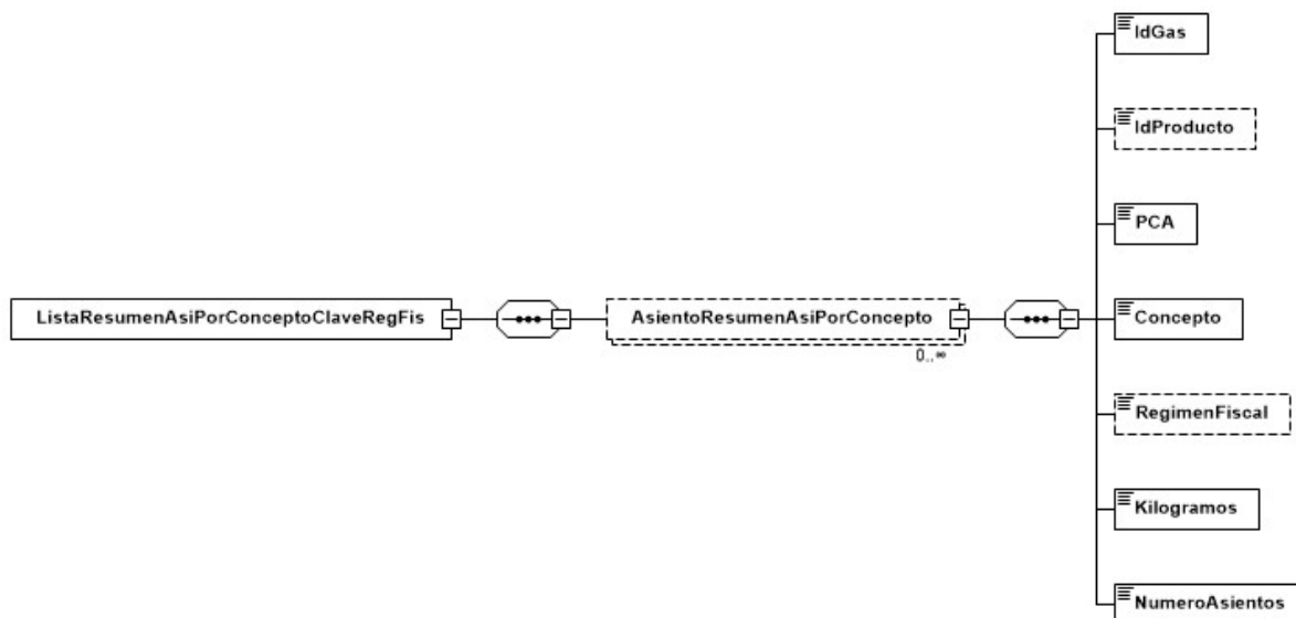
8. irudia. Laburpen datuak kontzeptuaren, gakoaren eta zerga araubidearen arabera
