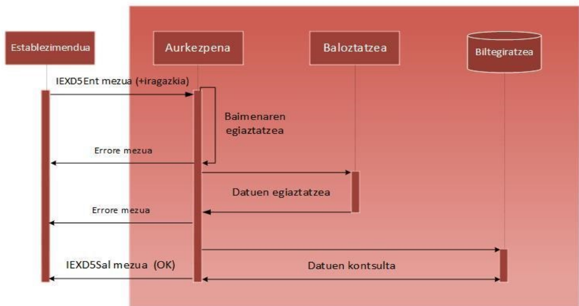
1. irudia. Kontsulta fluxua.
