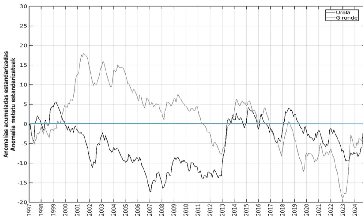
34. irudia. 1997-2024 bitartean Urolako eta Girondeko emariaren hileko datuetan izandako anomalia metatu estandarizatuak.
