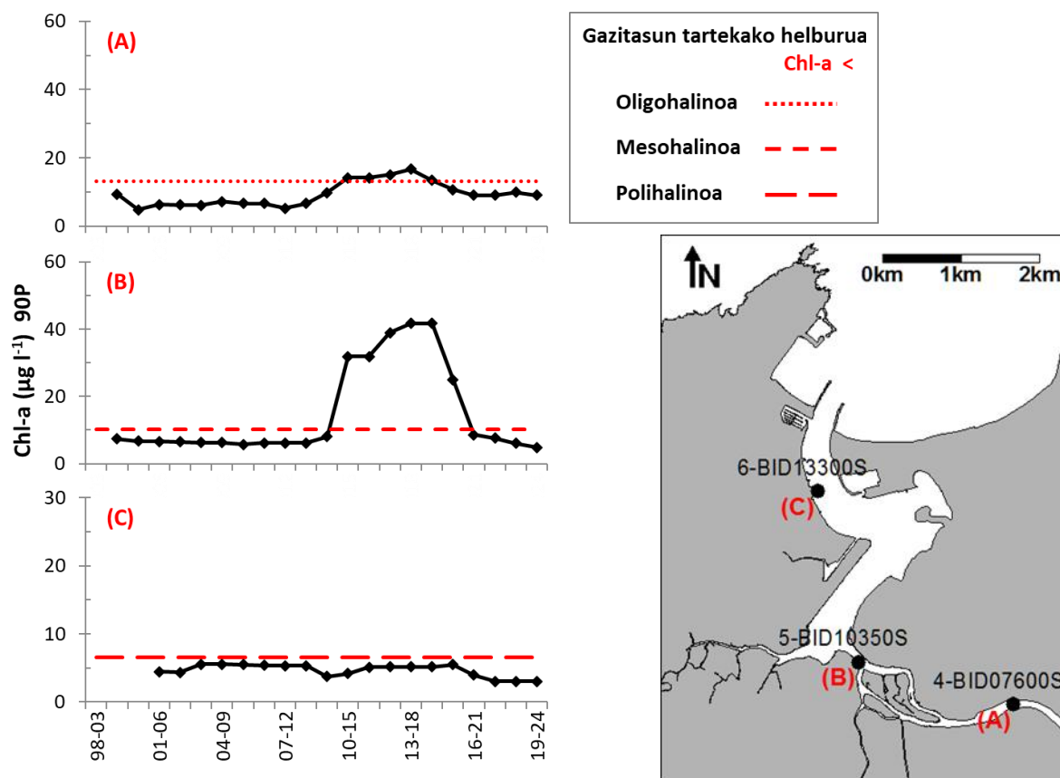
16. irudia. Klorofilaren kontzentrazioaren (Chl-a) 90. pertzentilaren bilakaera Bidasoa ibaiaren estuarioko hiru lagintze-puntutan: (A) BID07600S (goiko tarte); (B) BID10350S (erdiko tarte); (C) BID13300S (beheko tarte). Lerro gorriak gehiegizko biomasa fitoplanktonikoa adieraziko lukeen atalasea irudikatzen du. Ikus beheko aldea, polihalinao (C), irudikatzen duen irudiaren Y ardatzeko eskalaren aldaketa.
