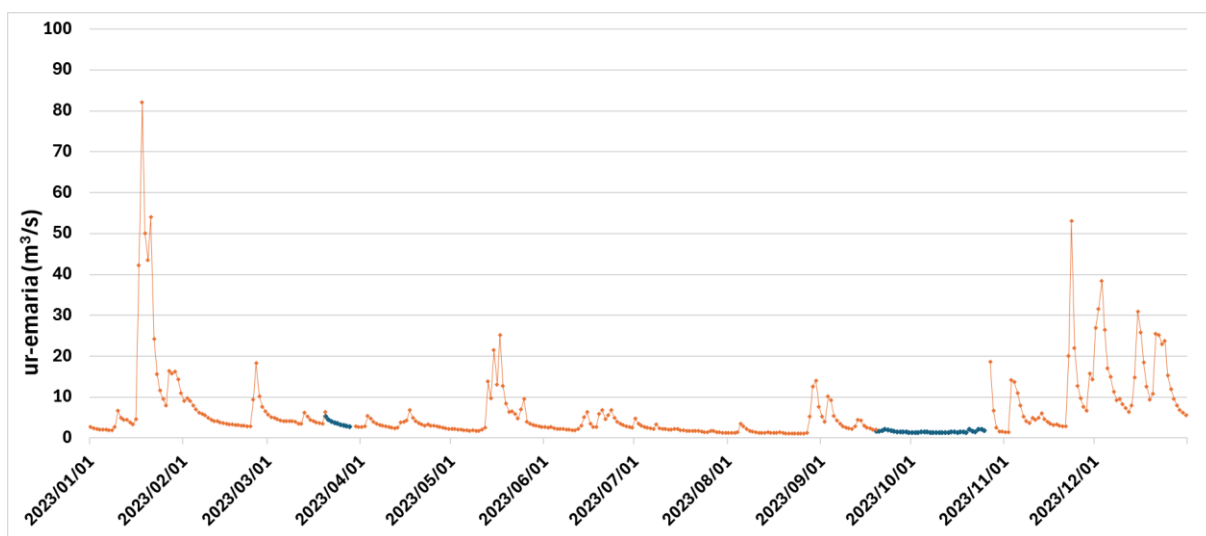
9. irudia. Urolaren emariaren bilakaera 2023. urterako ( \text{m}^3/\text{s} ). Neurtutako datuak (laranjaz) eta Debako emaritik abiatuta RMA erregresioarekin kalkulaturako datuak (urdinez).
