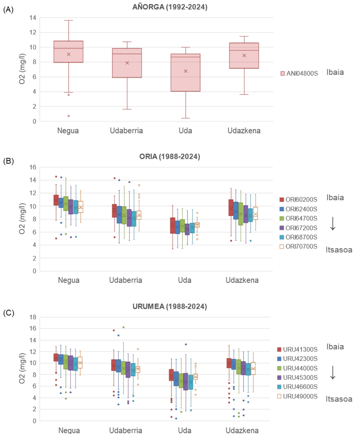
19. irudia. Oxigeno disolbatuari (O 2 ) buruzko estatistikoak ondorengo lagintze-puntuetan: (A) Añorga erreka; (B) Oria ibaiaren estuarioa; (C) Urumea ibaiaren estuarioa. Ikurrak: puntuak (balio atipikoak, outlier -ak); gurutzea (batezbesteko aritmetikoa); kutxa (25, 50 eta 75. pertzentilak); goi-bibotea (balio maximoa outlier -ak baztertuta), behe-bibotea (balio minimoa outlier -ak baztertuta). Neurketak berriki (2000ko hamarkadan) hasi ziren lagintze-puntuetan kolore gabeko kutxak ageri dira. ORI70700S eta URU49000S 2001.ean hasi ziren neurtzen.
