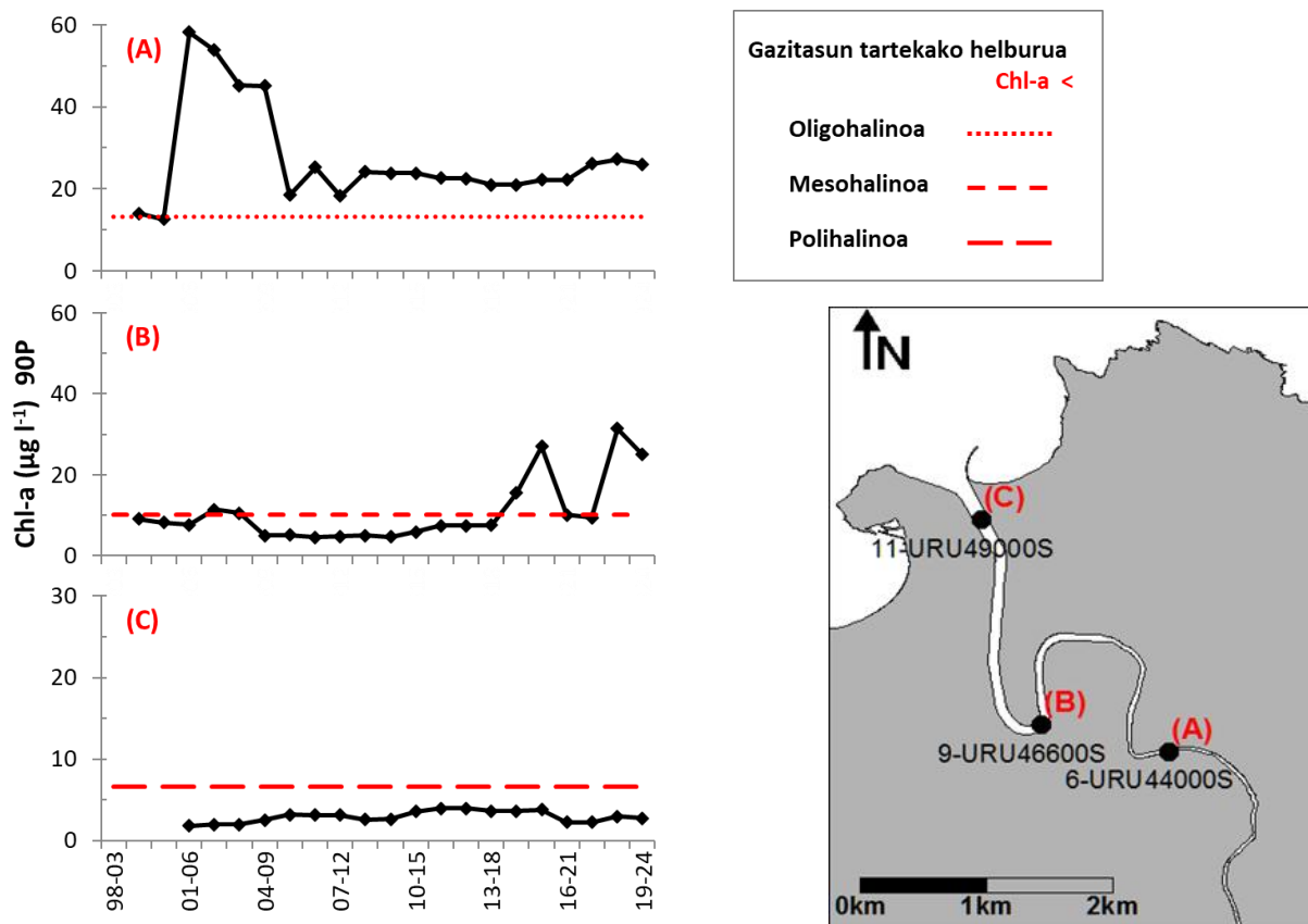
14. Irudia. Klorofilaren kontzentrazioaren (Chl-a) 90. pertzentilaren bilakaera Urumea ibaiaren estuarioko hiru lagintze-puntutan: URU44000S (goiko tartea); (B) URU46600S (erdiko tartea); (C) URU49000S (beheko tartea). Lerro gorriak gehiegizko biomasa fitoplanktonikoa adieraziko lukeen atalasea irudikatzen du. Ikus beheko aldea, polihalinoa (C), irudikatzen duen irudiaren Y ardatzeko eskalaren aldaketa.
