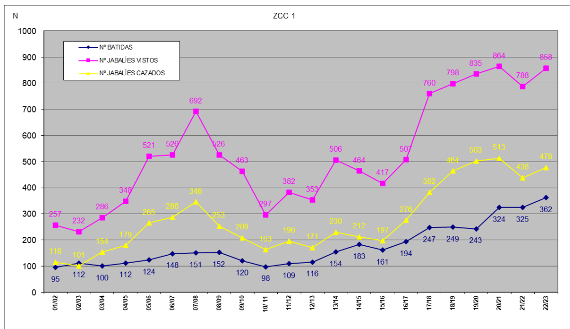
1. Irudia. Basurde ehizaren emaitza orokorrak 1 ZEEen.
