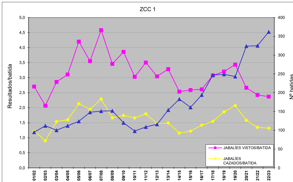
2. Irudia. Ugaritasun indizeen bilakaera 1 ZEEn.
