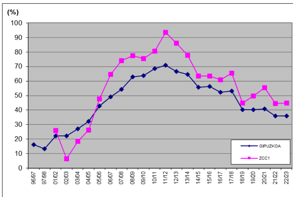
4. Irudia. Basurde uxaldietan orkatza agertzeko maiztasuna.
