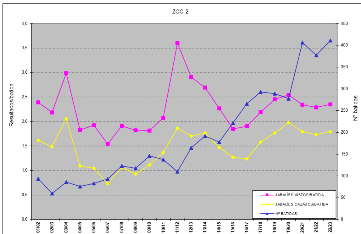
2. Irudia Ugaritasun indizeen bilakaera 2 ZEEn.
