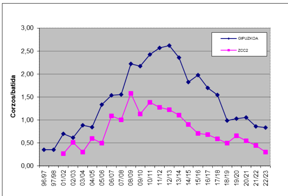
5. Irudia Basurde uxaldi bakoitzean ikusitako orkatzak.
