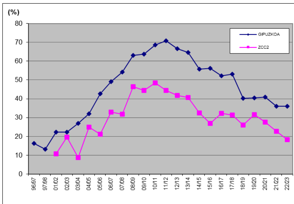
4. Irudia Basurde uxaldietan orkatza agertzeko maiztasuna.
