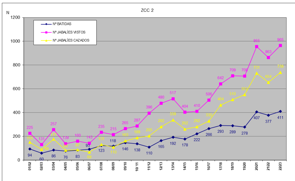
1. Irudia Basurde ehizaren emaitza orokorrak 2 ZEEen.
