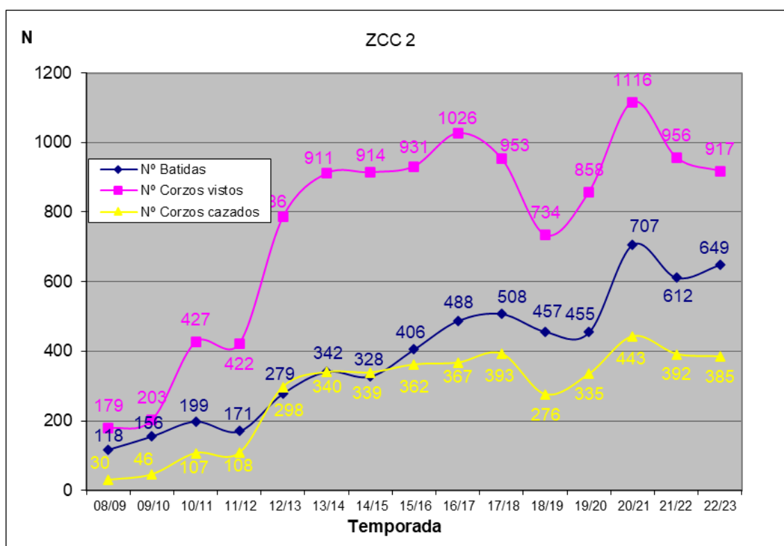
3. Irudia Orkatz ehizaren emaitzak 2 Zainpeko Ehiza Eremuko ehiza larriko uxaldietan.
